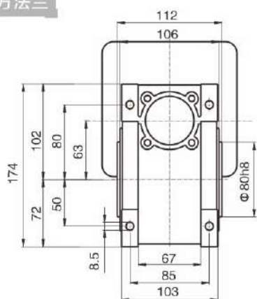
方法兰
