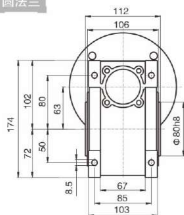
圆法兰
