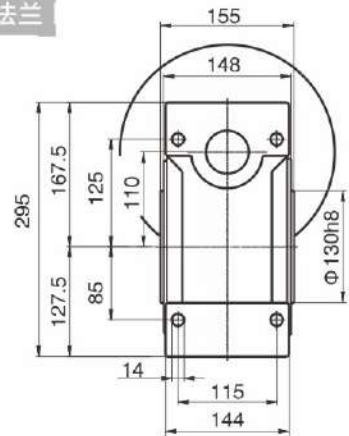
圆法兰
