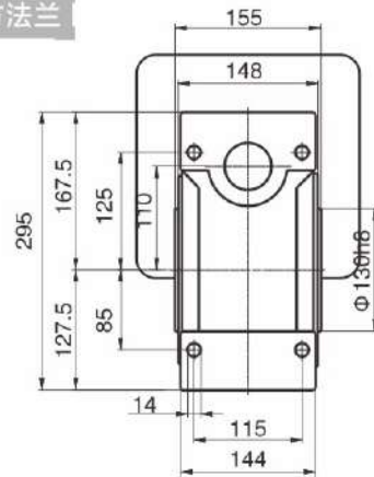
方法兰
