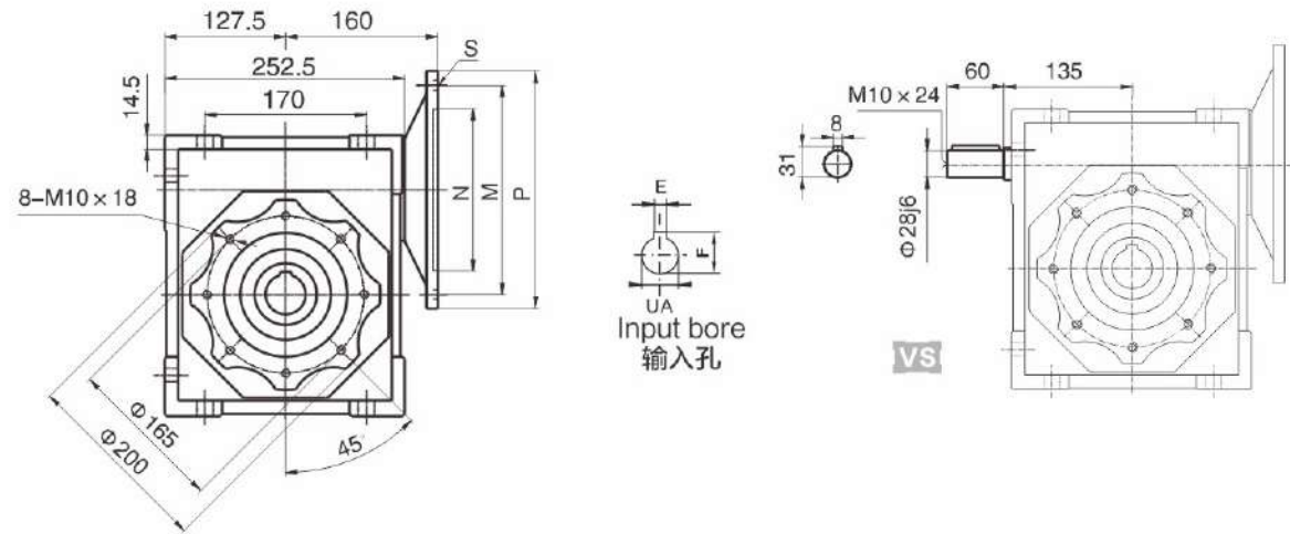
圆法兰
